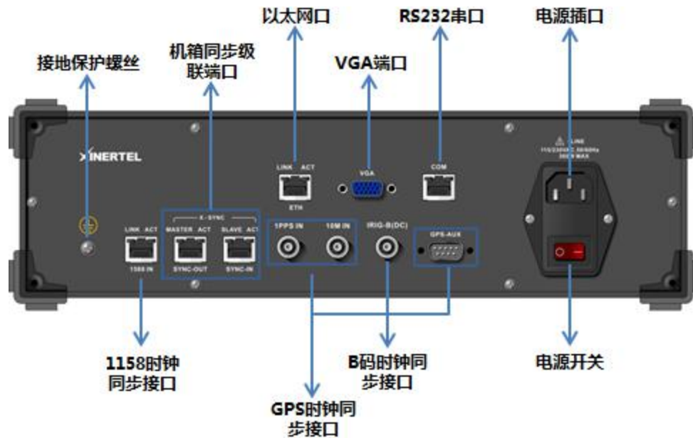
图 2 信而泰 BigTao210 后面板示意图
